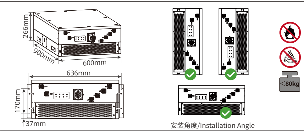
安装角度/Installation Angle BTH10INT0004
